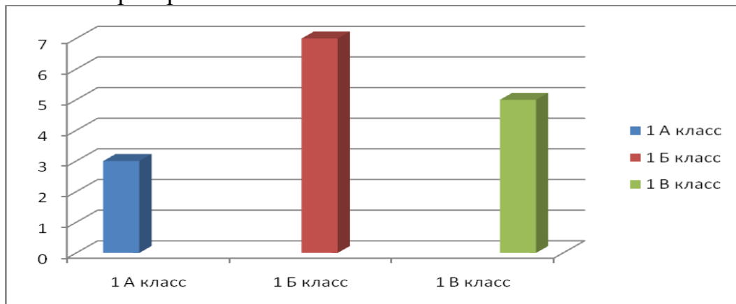
Гистограмма данных
