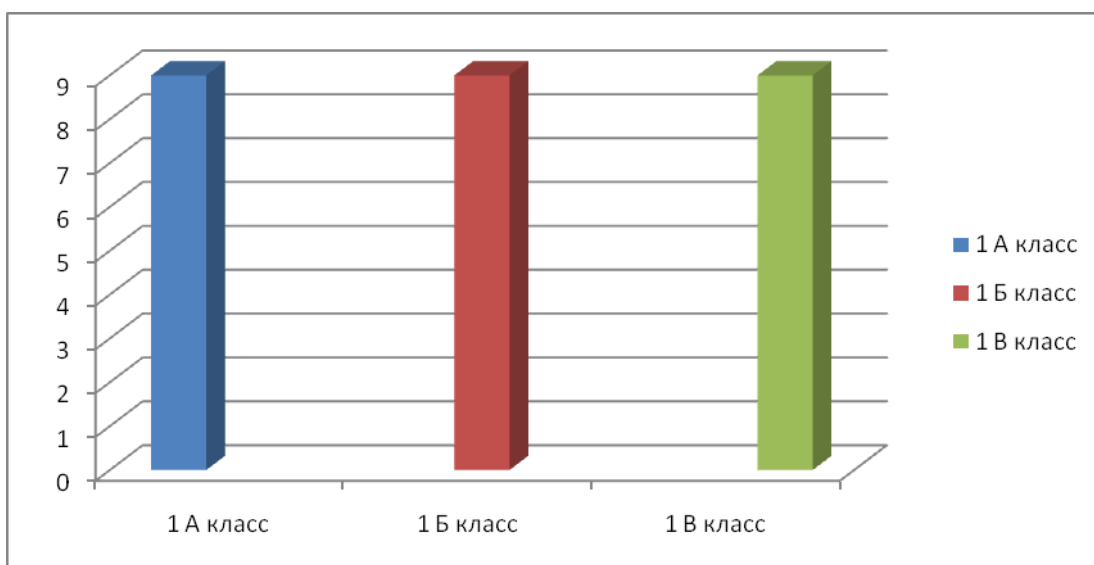
Гистограмма данных
